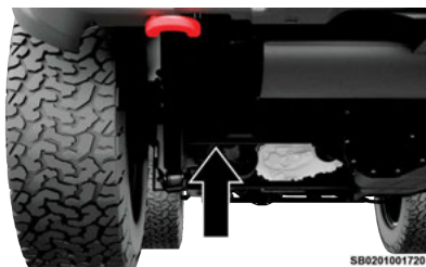
リヤ側ジャッキ位置
