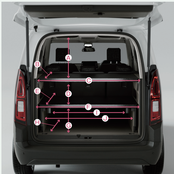
5人乗りモデル 寸法
